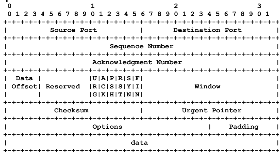
Рисунок 3. Формат заголовка TCP
