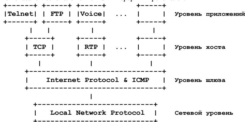
Рисунок 2. Отношения между протоколами
