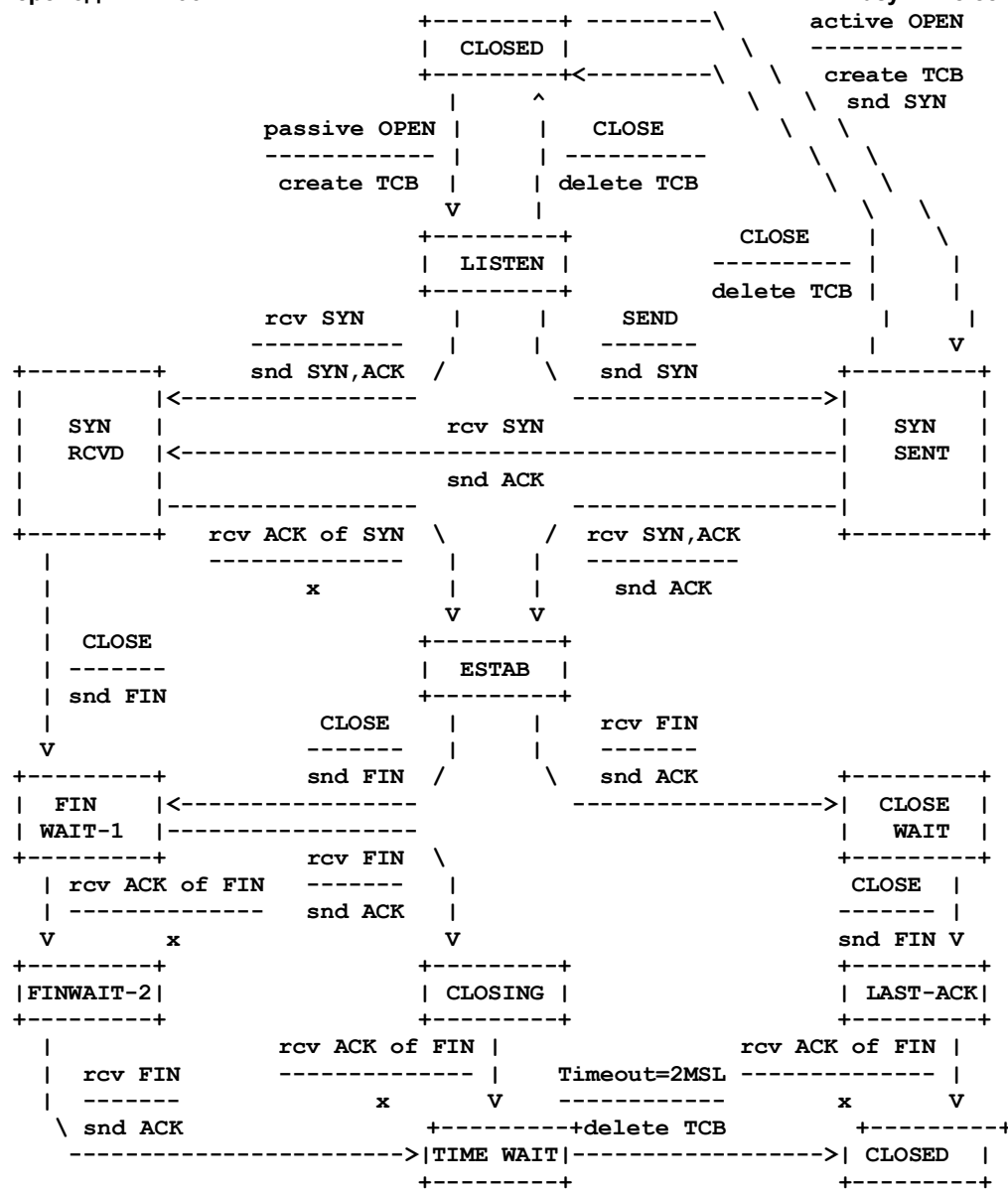
Рисунок 6. Состояния соединений TCP 5
